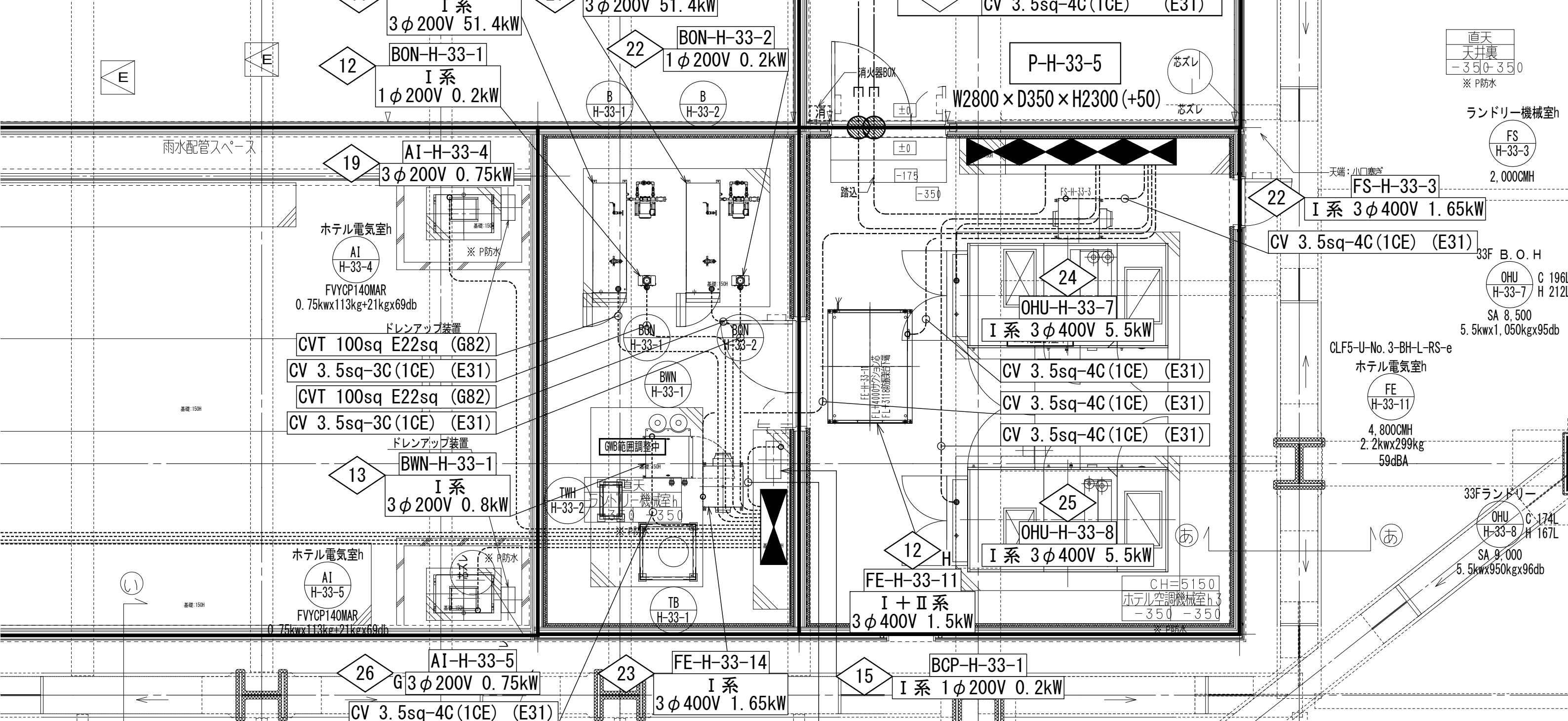
P-H-33-6 負荷リスト
